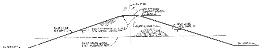
SECTION 1 SCALE: 1"=20'
