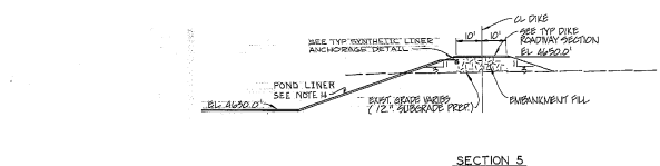
SECTION 5 SCALE: 1"=20'
