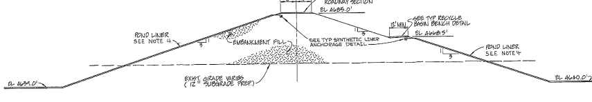
SECTION 3 SCALE: 1"=20'
