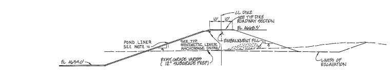
SECTION 4 SCALE: 1"=20'
