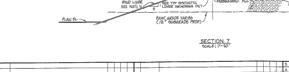
SECTION 7 SCALE: 1"=20'
