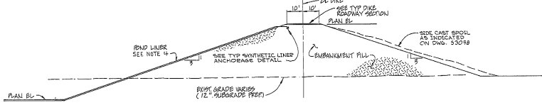
SECTION 2 SCALE: 1"=20'
