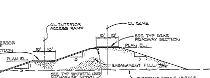
SECTION 8 SCALE: 1"=20'
