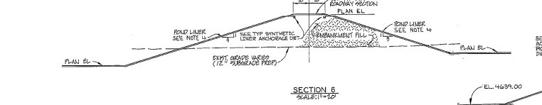
SECTION 6 SCALE: 1"=20'
