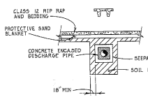
SECTION 4 SCALE: 1/4\"/>
